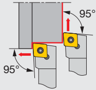
Cutting edge style L
