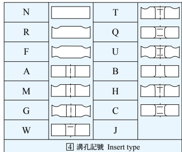
4 溝孔記號 Insert type
