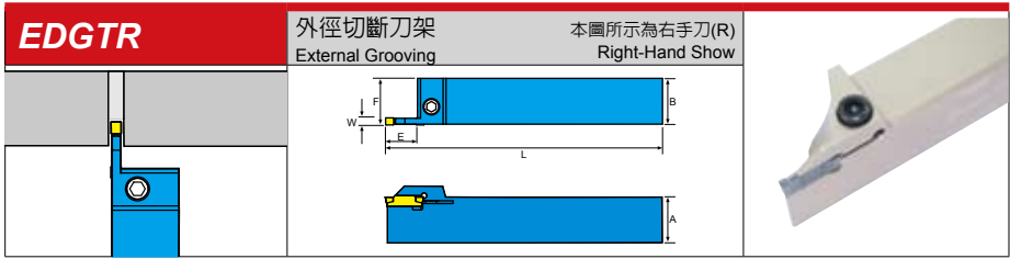
外徑切斷刀架系列 / Tool Holders for External Deep Turning
