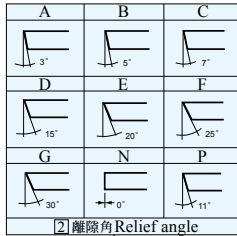
2 離隙角 Relief angle
